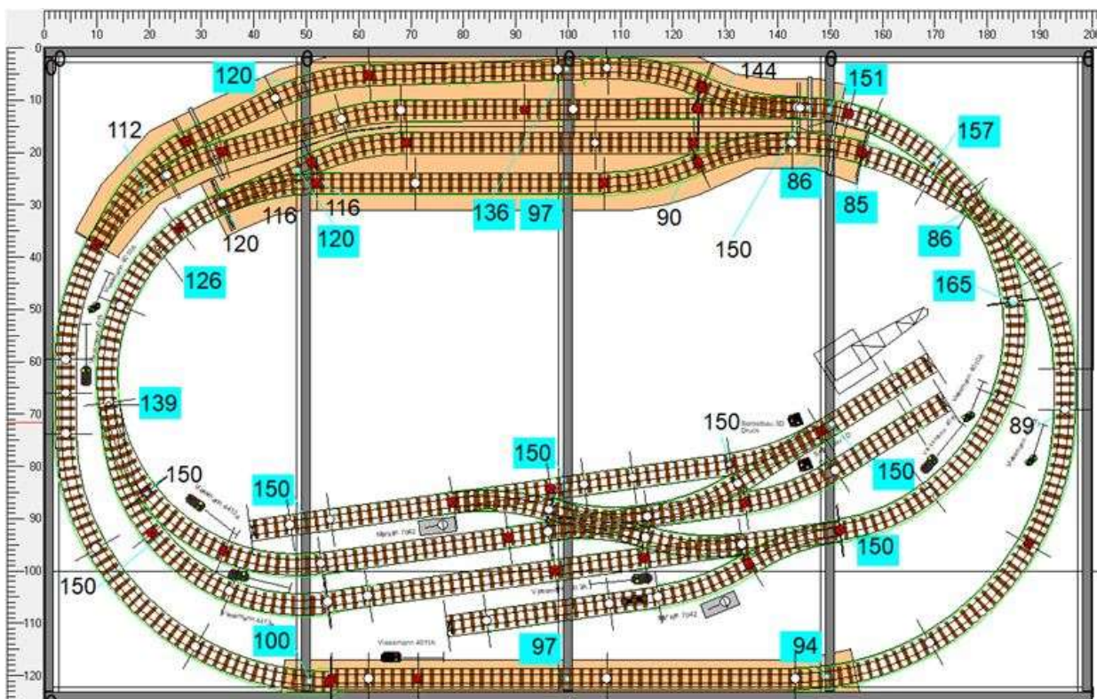
Bild 1: Gleisplan einer kleineren Modelleisenbahnanlage
