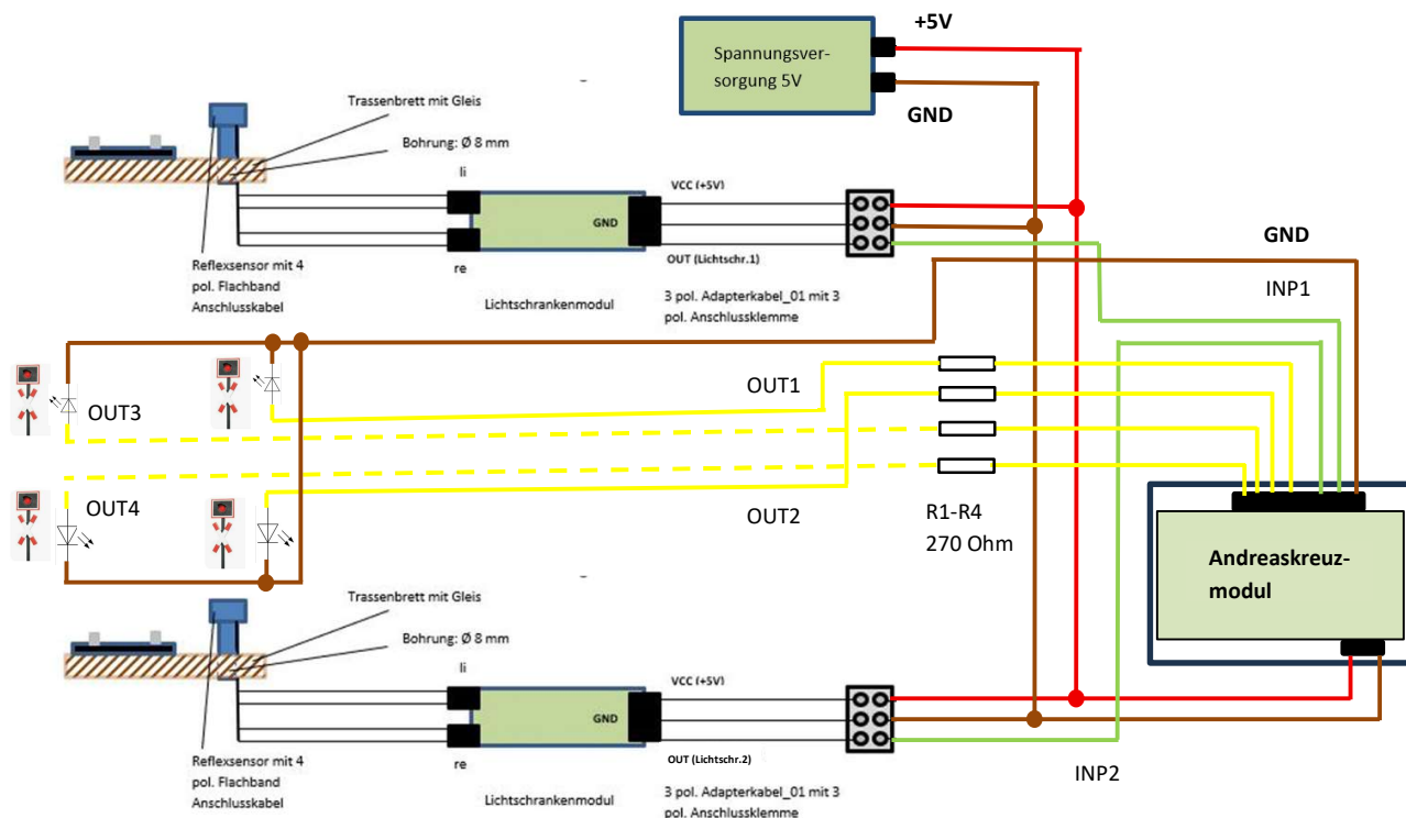
Bild 6.2.1: Anschluss – Andreaskreuzmodul mit 5V Versorgung und 2 Reflex-Lichtschrankenmodulen
